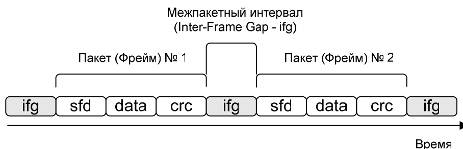
Рисунок 20-1. Передача фреймов
