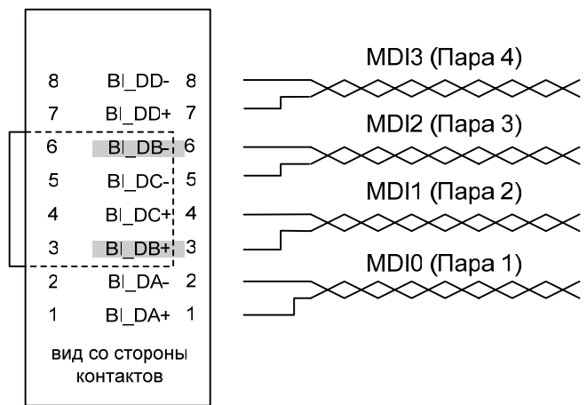
Рисунок 17-1. Неправильное подключение.
