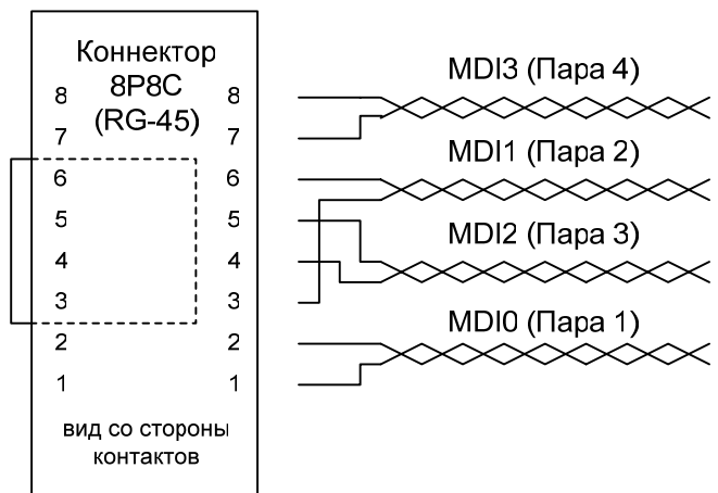
Рисунок 17-2. Правильное подключение.
